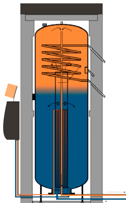
Sezione Coax 390
